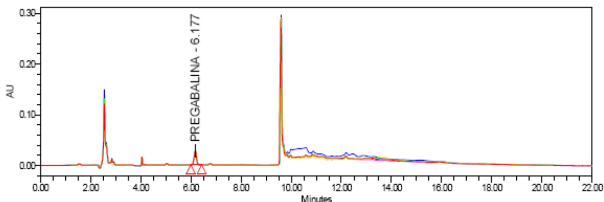
Grafico 3: Cromatograma de la solución estándar
