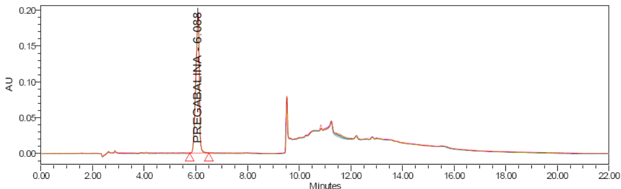
Gráfico 2: Cromatograma de la solución muestra
