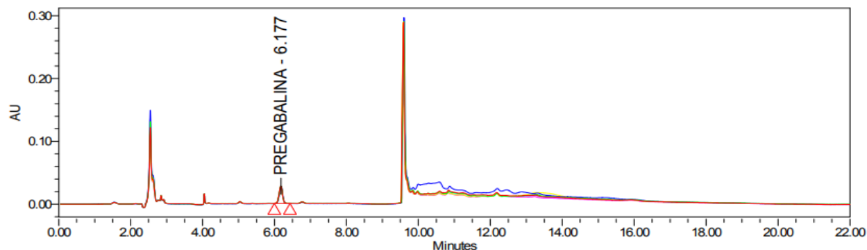
Gráfico 4: Cromatograma de la solución muestra
